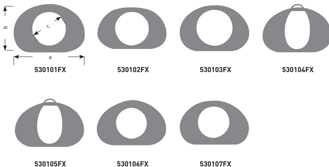
530101FX large, for adults / 17 cm, a/b/c = 29/19/16 mm groß, für Erwachsene / 17 cm, a/b/c = 29/19/16 mm
